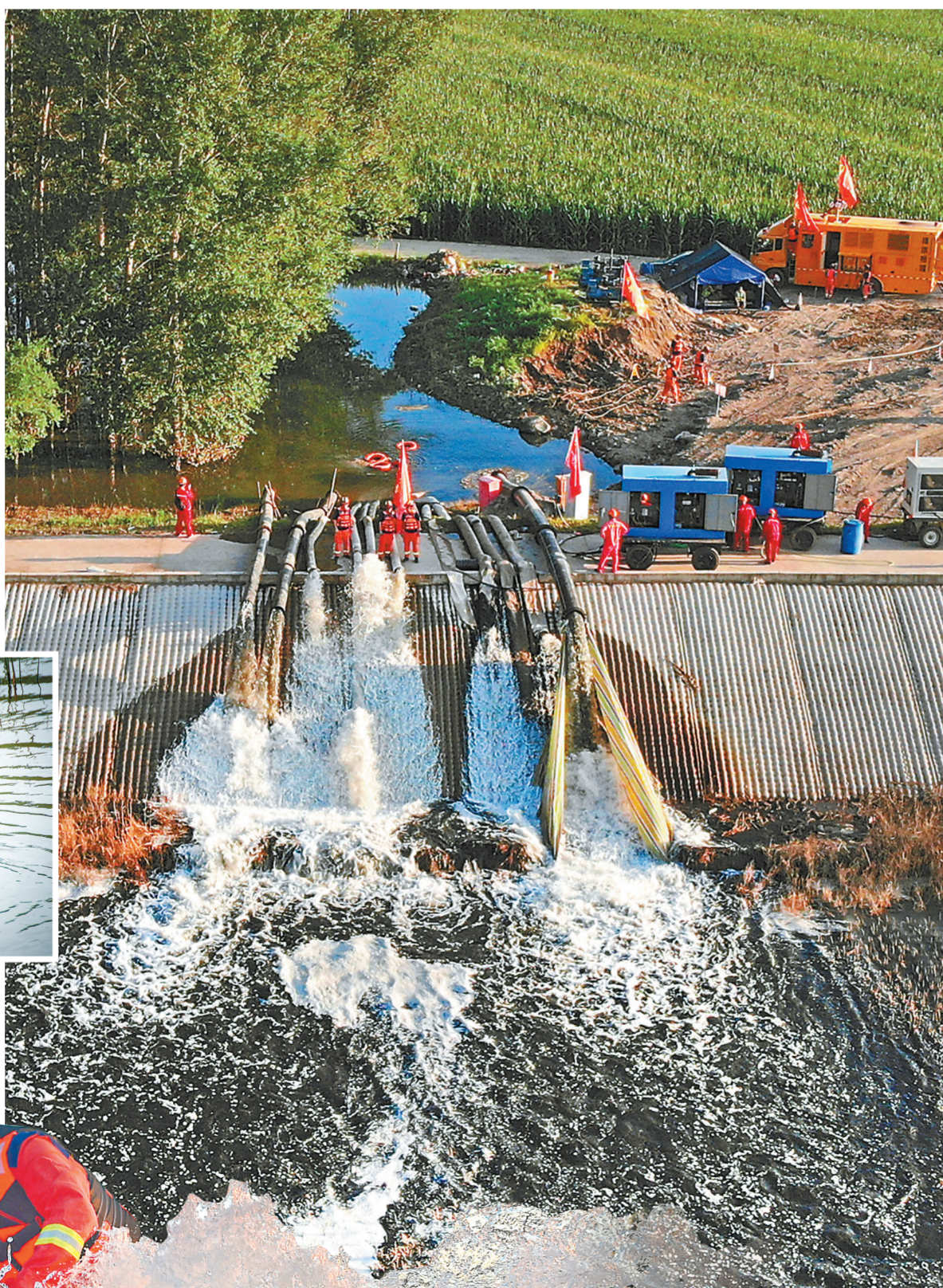
吉林省松原市扶余市双城区拉林河大桥附近7号点排涝现场,胜利油田救援队将农田积水排进河道。
